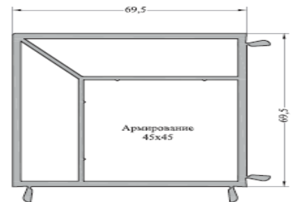
Профиль угловой 90/70 с уплотнением арт.10405070.25
