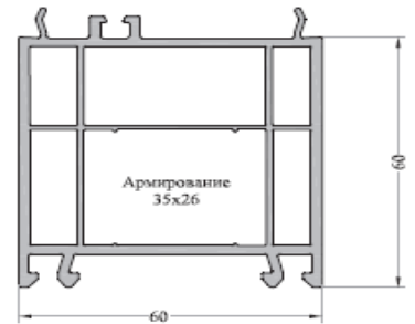
Профиль доборный 60/60 с уплотнением ТЭП арт.10106060.16
