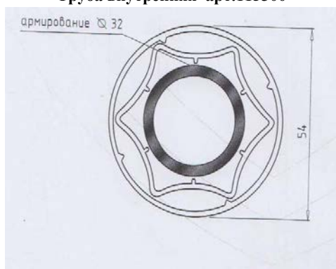
Труба внутренняя арт.115300
