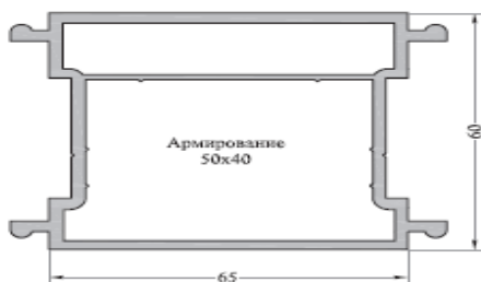
Профиль соединительный 65/60 арт.10105065
