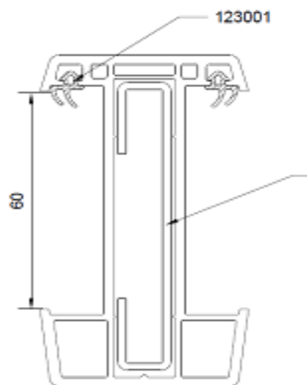
Профиль статического усилителя 60 мм арт.666100
