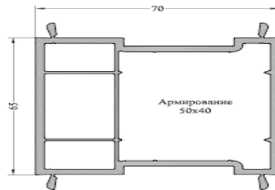
Профиль соединительный 65/70 арт.10405065
