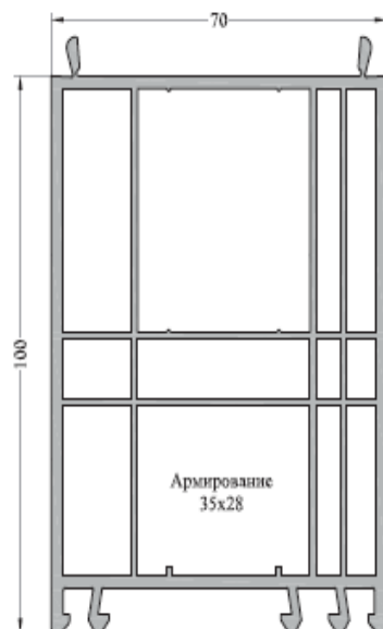
Профиль доборный 100/70 с уплотнителем арт10406100.25
