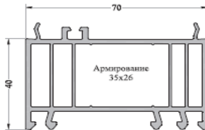
Профиль доборный 40/70 с уплотнением ТЭП арт.10406070.16
