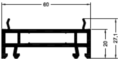
Профиль доборный 20/60 с уплотнением арт.10106020.25
