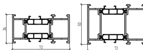
Профили уширителя
