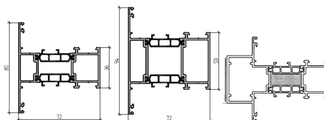
Профили импоста
