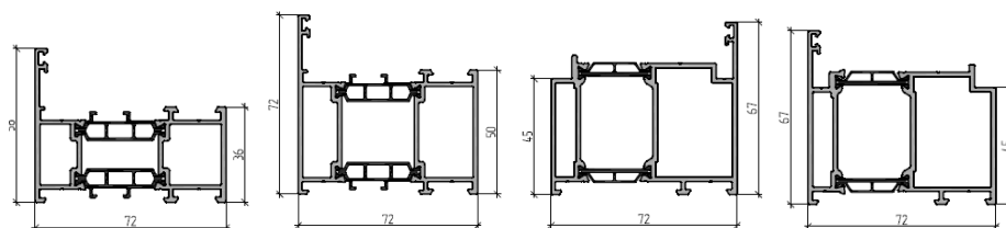
Профили рамы
