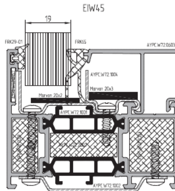
Использование стального усиливающего элемента без дополнительной обработки профилей и штапиков
