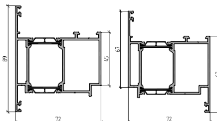
Профили створки
