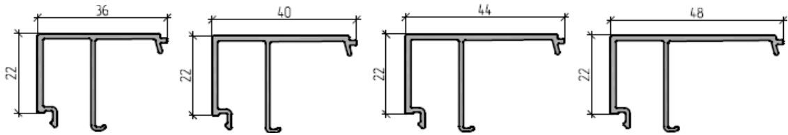
Оригинальные профили штапиков W72 FR
